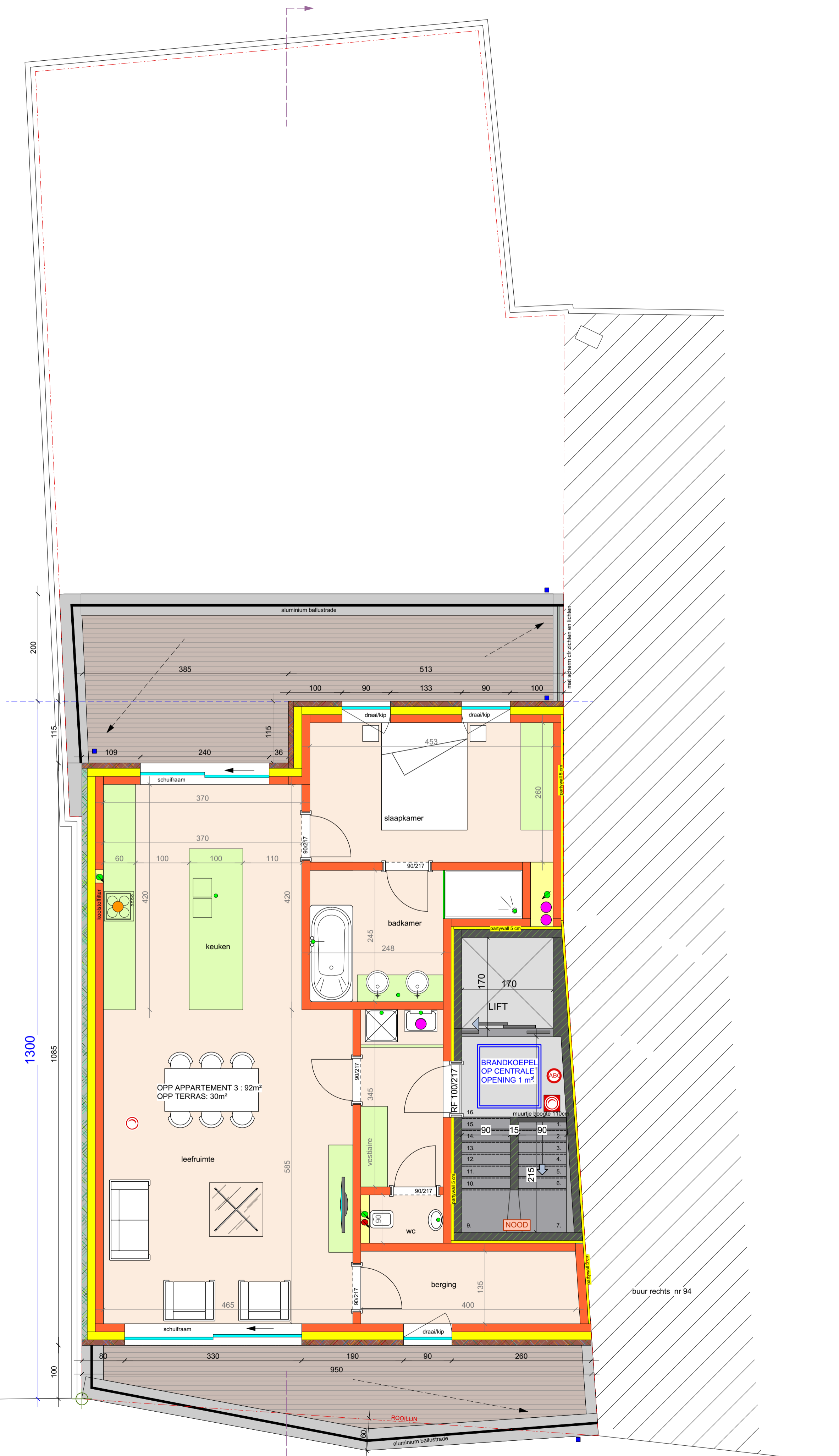
PLAN VERDIEPING 3 schaal 1/50
