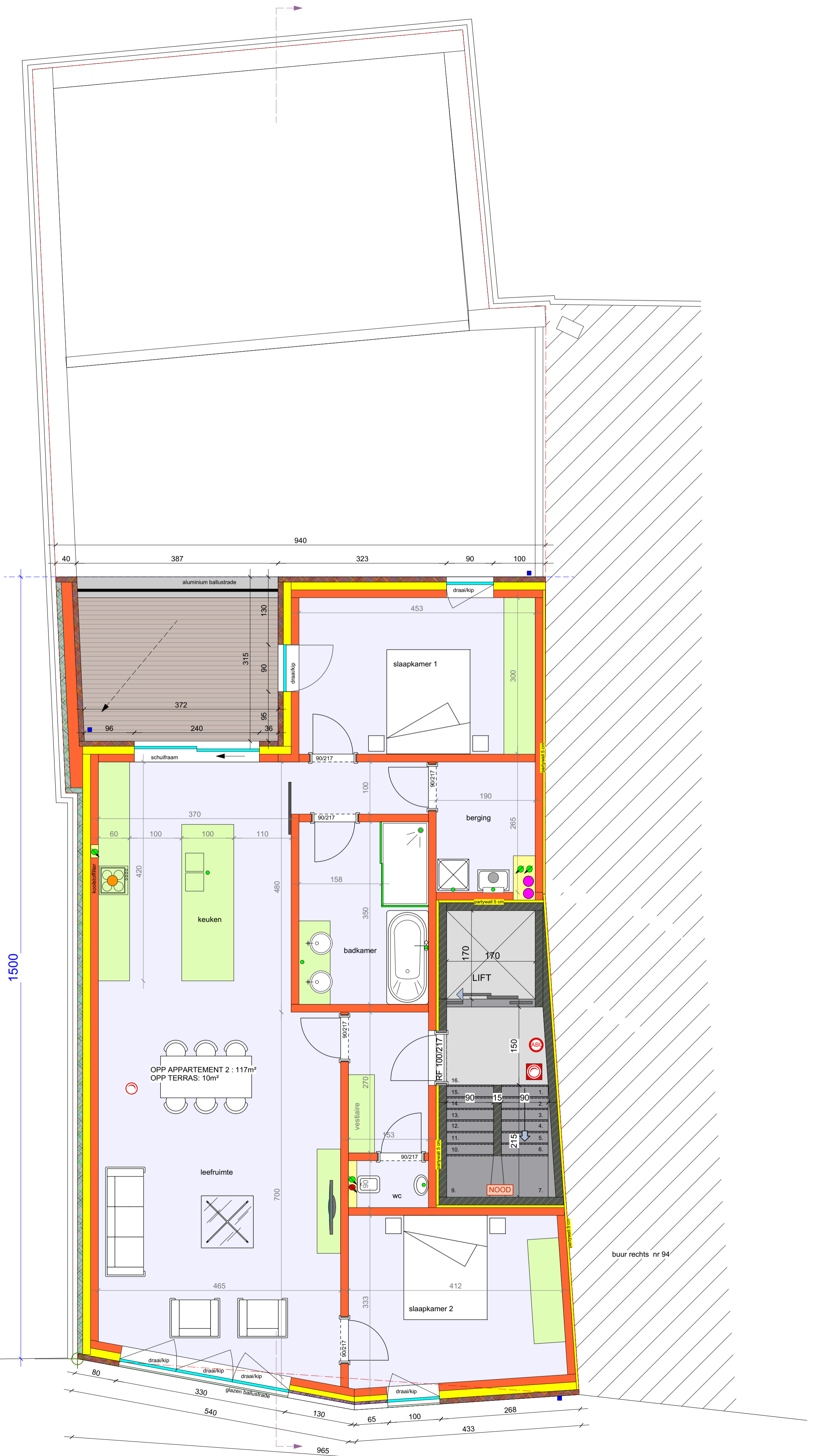
PLAN VERDIEPING 2 schaal 1/50
