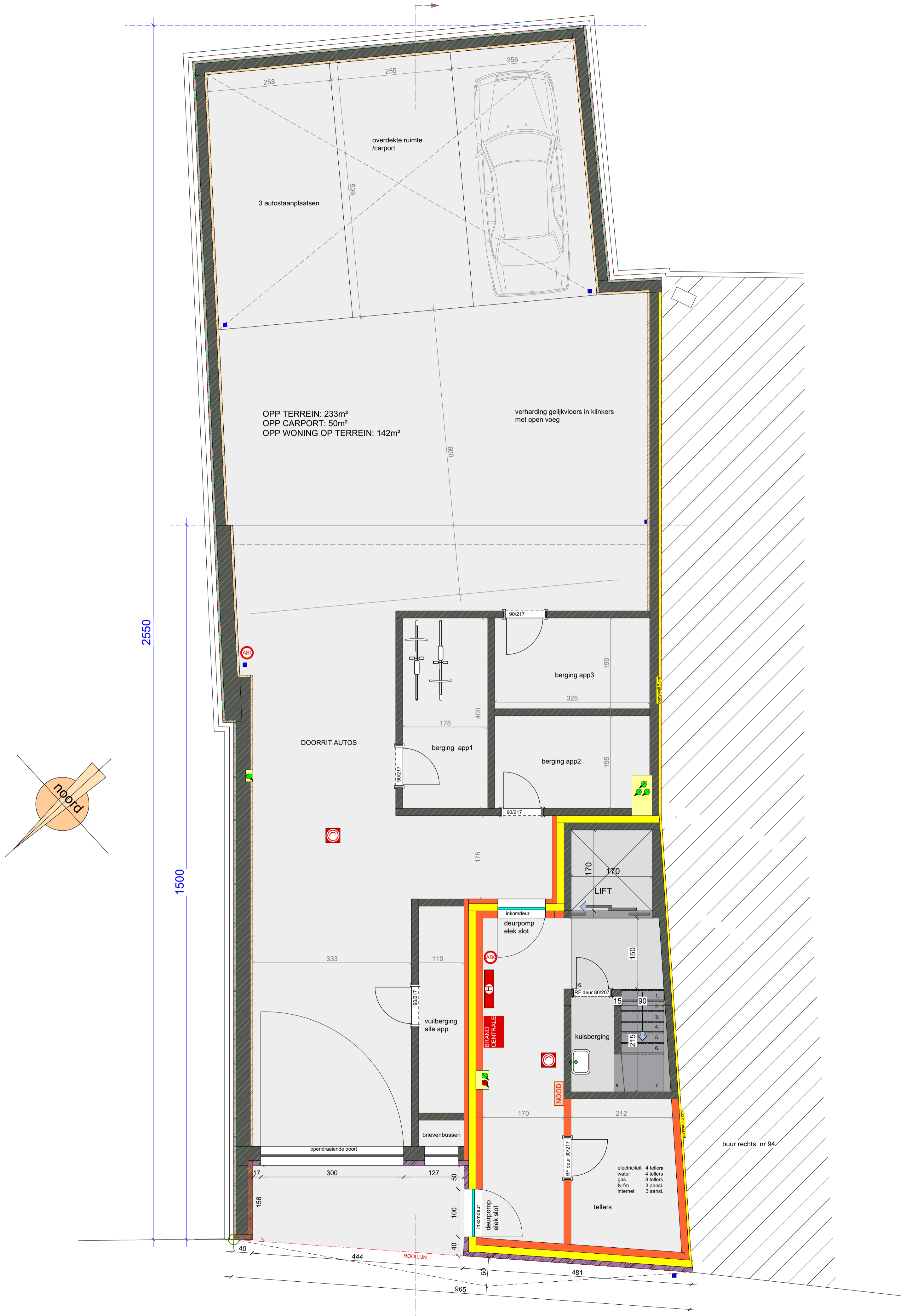
GELIJKVLOERS schaal 1/50
